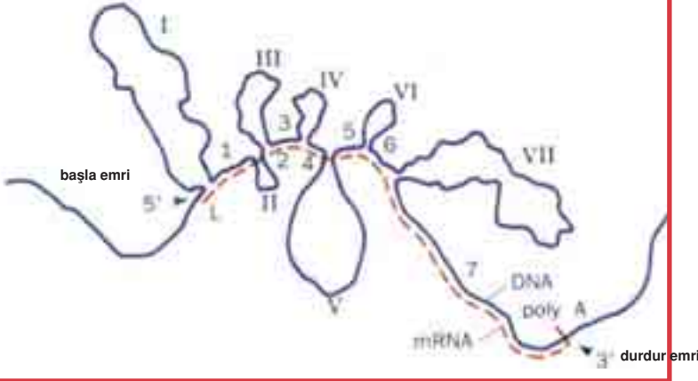
(Şekil 3.4) DNA'nın akıllı gösterip mesajcı RNA'ya yalnızca gerekli bilgileri sunması. I,II,III,IV,V,VI,VII ile işaretlenmiş bölüm okunması istenmeyen bilgi içerir. Bu yüzden dışarı doğru kıvrılarak DNA bu bölgenin kopyalanmasını engeller. 1,2,3,4,5,6,7,8 ile işaretlenen gerekli bilgi mesajcı RNA'ya sunulur. Karbon, hidrojen ve fosfat gibi şuursuz atomların bu akıllı gösteremeyecekleri, bu akıllı o bilgileri oraya yazan, okutan ve hayata geçiren Allah'a ait olduğu çok açıktır.
