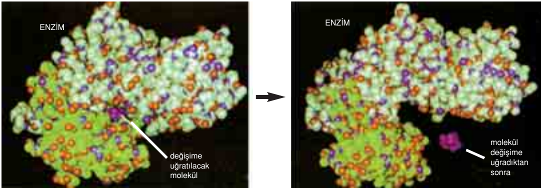
(Şekil 5.4) Bir enzim(heksokinaz) ve etki ettiği madde arasındaki üç boyutlu kusursuz uyumu gösteren şekil. Heksokinaz enzimi ATP molekülünü ADP'ye, ADP'yi ATP'ye çevirir. Birinci karede enzim değişime uğrattığı molekül üzerine bir kalıp gibi kapanır. İkinci karede enzimin parçaları birbirlerinden ayrılır ve molekül değişime uğramış bir şekilde ortama bırakılır.
