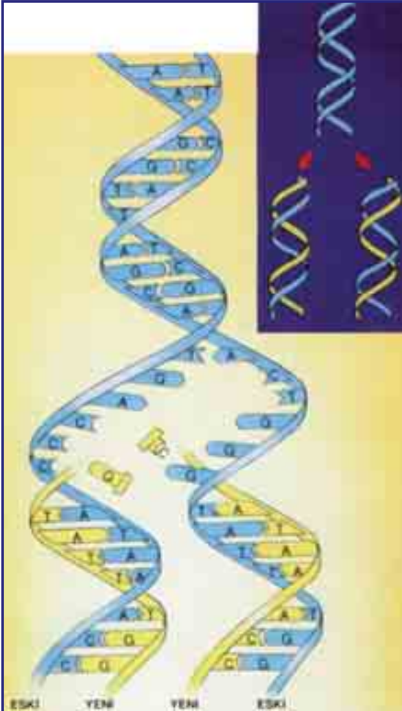
(Şekil 2.7) DNA sarmalının eşlenmesi. Sarmal birçok enzimin yardımıyla önce bir fermuar gibi ortadan ikiye ayrılır. Daha sonra her parçanın eşleniği olan nükleotidler ortamdand temin edilerek yarım parçaya yapıştırılır. Böylece birbirinin kopyası iki yeni DNA sarmalı oluşur.
